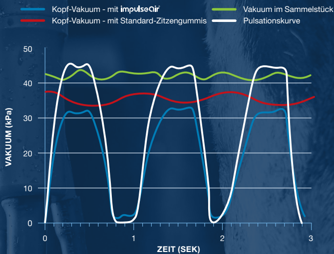
Diagramm zeigt verminderte Vakuumaktivität an der Zitze mit impulseAir .
